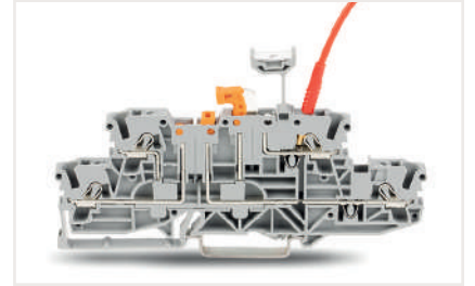
Çift katlı, çift ayrılmalı klemens (2002-2951), grup işaret taşıyıcısı (2002-160) bir köprü kontak yuvası ve test fişi (210-136) içine yerleştirilmiştir.
