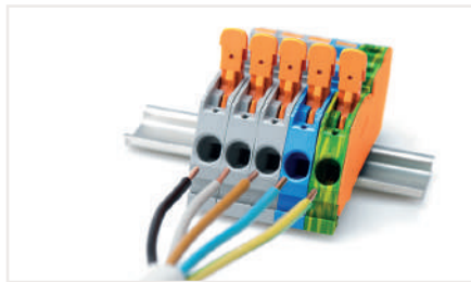
Kollu klemensler saha kabloları bağlantıları için idealdir.
