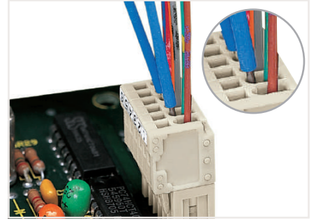
1 mm Ø test pini (Ürün No. 735-500) ile test, kontakta dokununuz.
