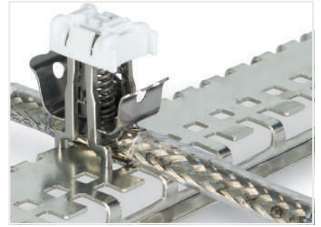
Ekran sıkıştırma modül kontakları ekran iletkeni ve özel yarıklı DIN rayı (790-145). Lütfen rayın altındaki ara modülü (790-144) kullanın.
