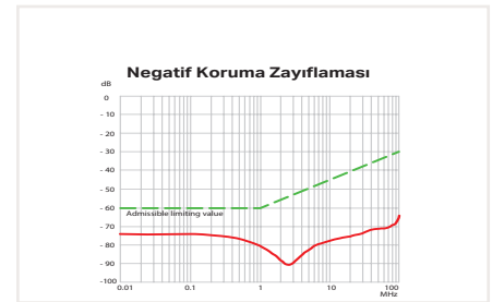
Blendaj bağlantı sistemi oldukça etkilidir çünkü sıkıştırma ünitesi kabloların blendajsız kısmına çok yaklaştırılabılır.
