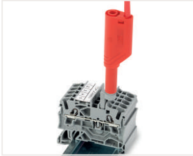
4 mm Ø fişler için test fiş adaptörü (2009-174, CAT I) - 2000 ile 2016 Serisi ile uyumlu
